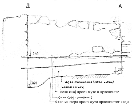
Западни профил сонде 6
